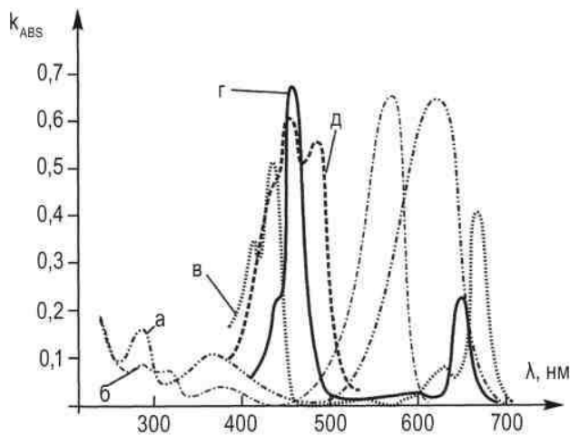
Рисунок 4 – Спектральні залежності відносних показників поглинання пігментів фітопланктону k_{ABS} від довжини хвилі \lambda
