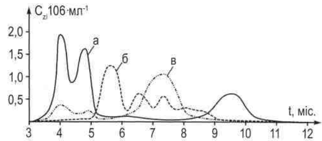
Рисунок 5 – Сезонні зміни співвідношень об'ємних концентрацій C_{zi} між різними групами фітопланктону: а – діатомові, б – зелені, в – синьо-зелені водорості
