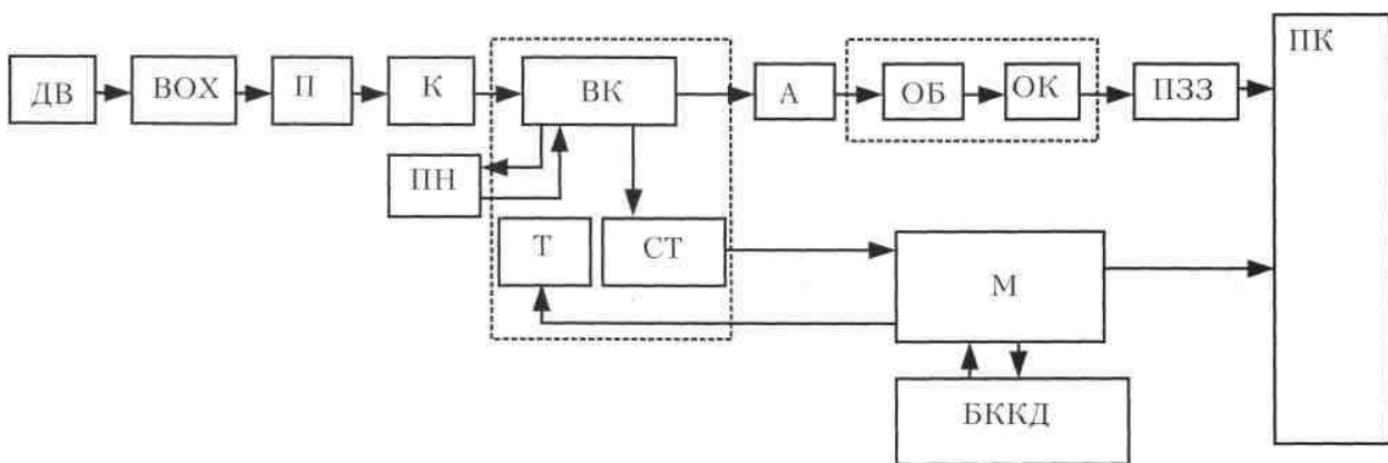
Рисунок 3 – Структурна схема засобу контролю стану водних об'єктів
