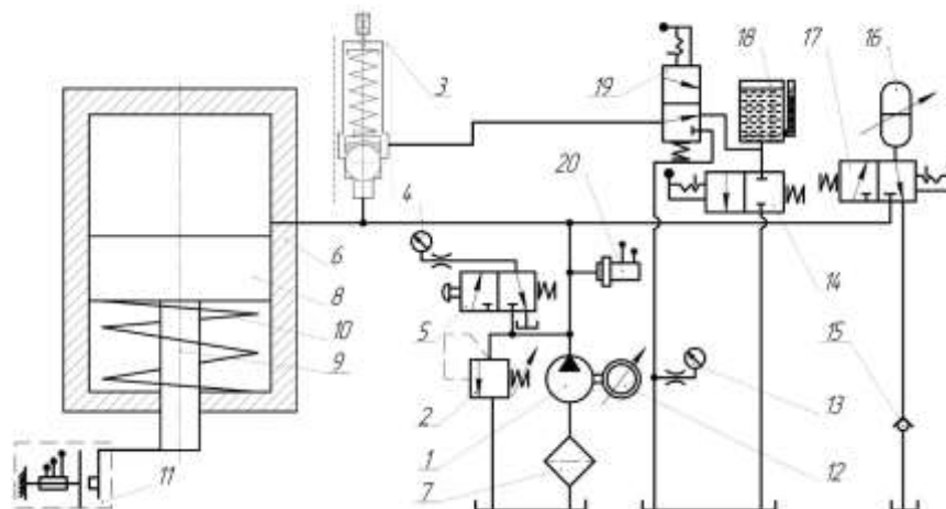
Рисунок 1 – Гідрокінематична схема експериментального стенду
