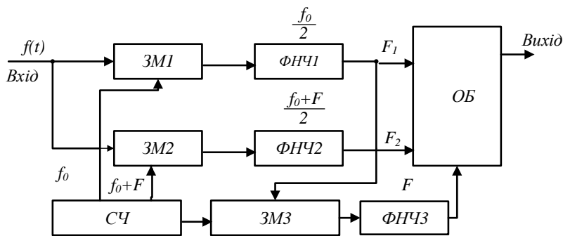
Рисунок 2. Структурна схема ідентифікатора з двократним перетворенням частоти
