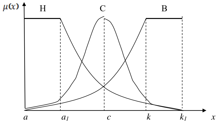
Рисунок 2 – Загальний вигляд функції належності трьох нечітких термів для показників x_{ij} [6]
