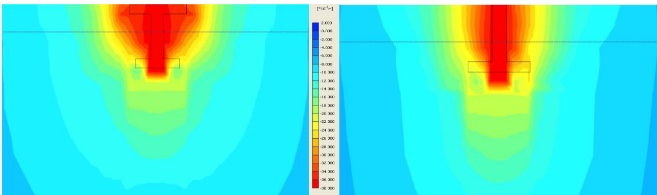
Рисунок 1 – Вертикальні деформації ґрунтового півпростору для варіанту розташування банкет в рівні поверхні ґрунту (а) та в рівні підшви фундаменту (б)
