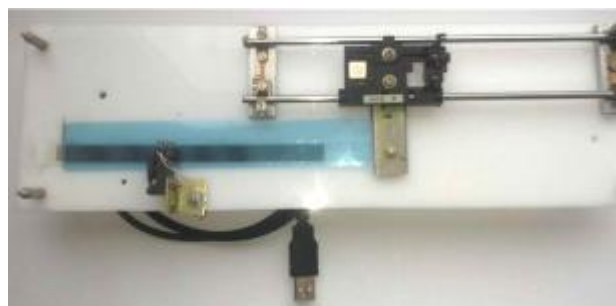
Рис. 2. Загальний вигляд діючої моделі сенсора лінійних переміщень на муаровому ефекті
