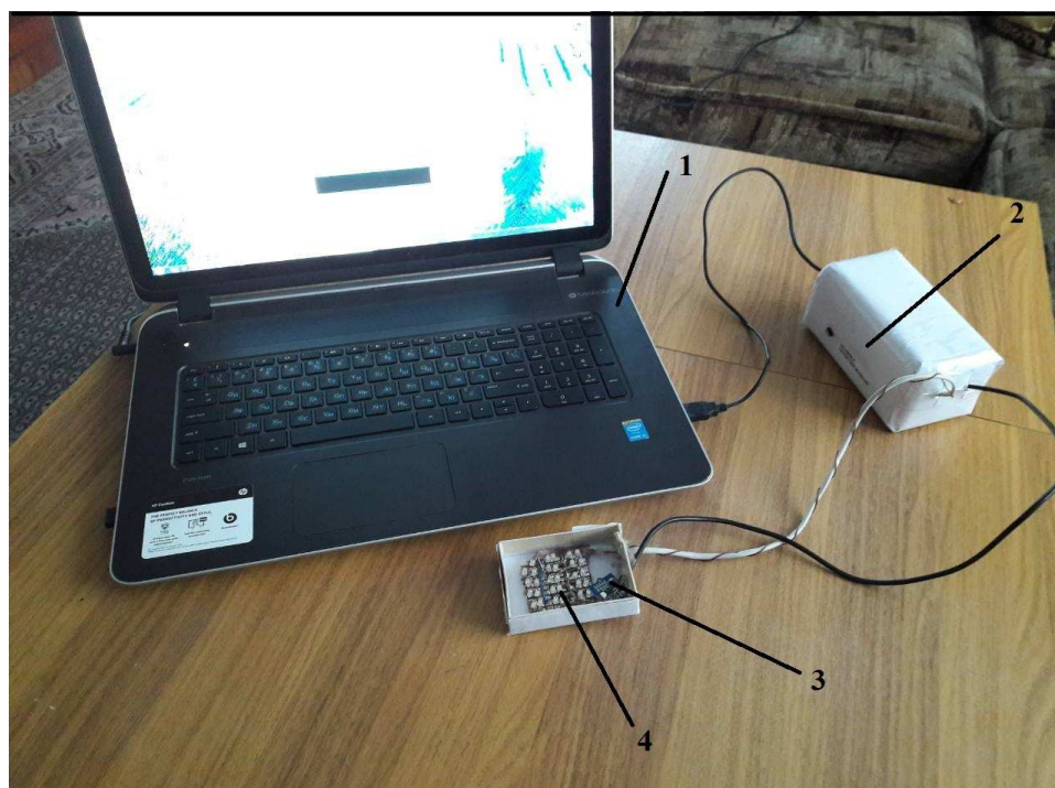
Рисунок 8 - Загальний вигляд дослідного зразка системи фізіотерапії. 1 - персональний комп'ютер з робочою програмою, 2 - мікроконтролер з елементами перетворювання вхідного сигналу, 3 - фотоприймач, 4 - напівпровідникова матриця з випромінювачами
