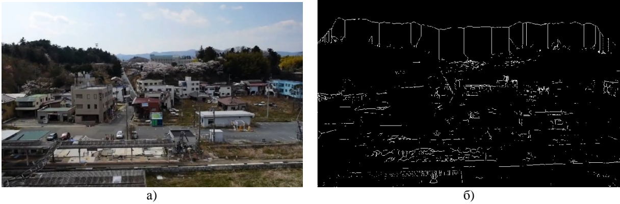
Рис. 7. Скелетування зображення
