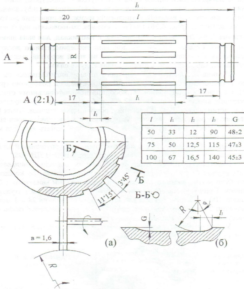
Рисунок 1 — Вал газового підвісу з повздожніми канавками
