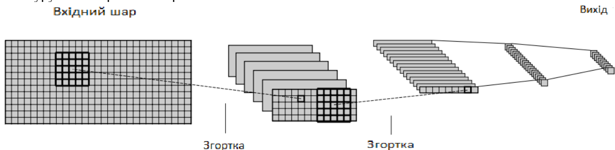
Рис. 2. Архітектура згорткової нейронної мережі для розпізнавання мовця
