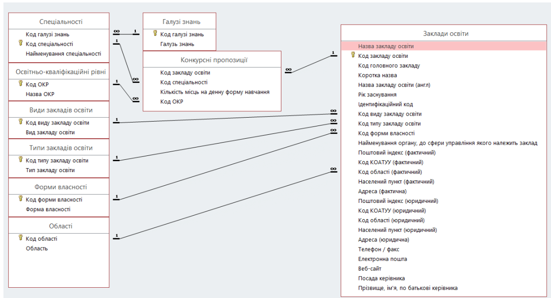
Рисунок 1 – Схема даних
