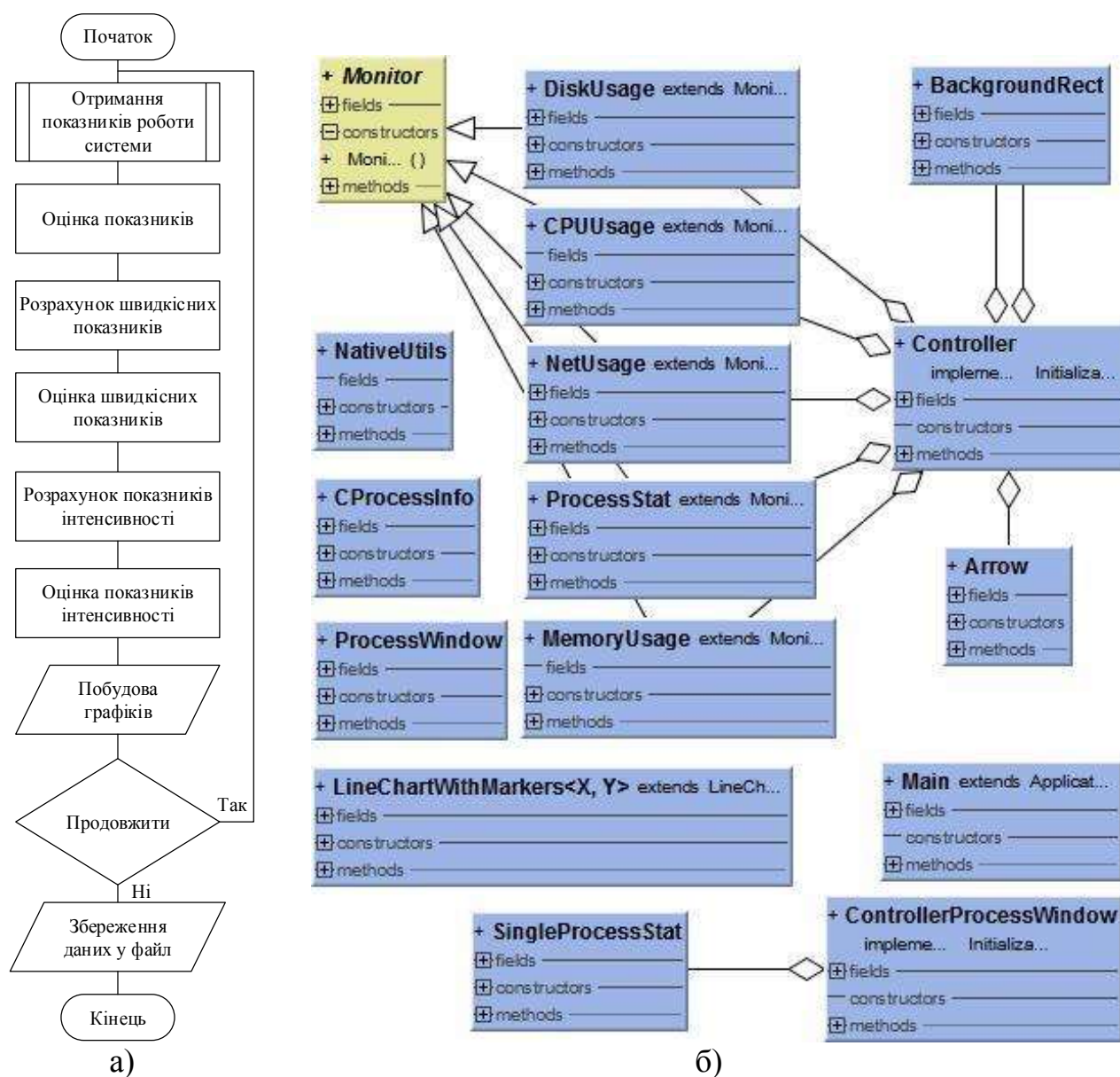
Рисунк 3 – Блок-схема алгоритму програми (а) та UML діаграма класів програмного додатку
