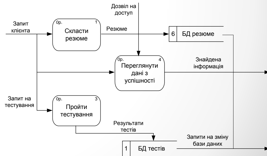
Діаграма DFD
