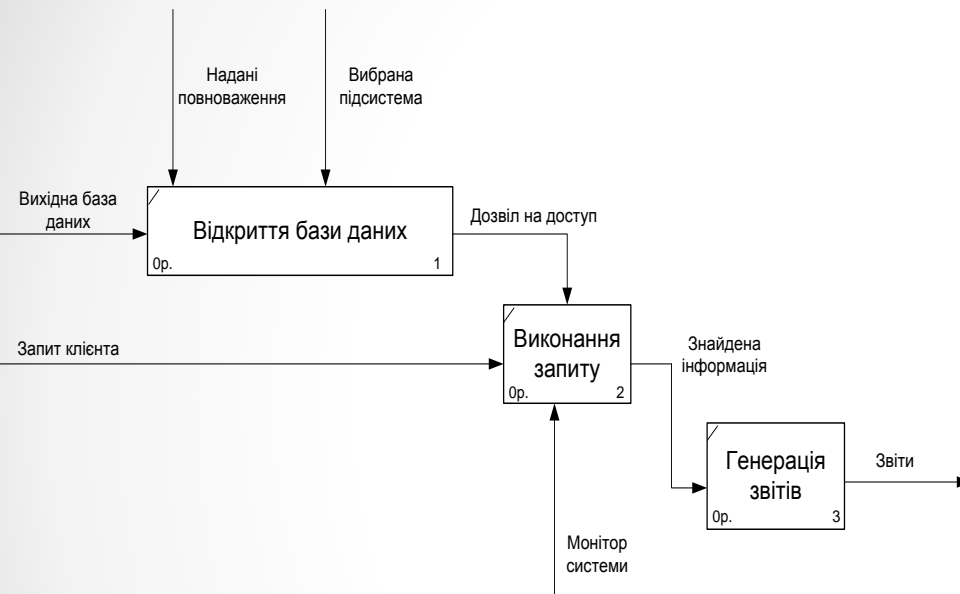
Діаграма IDEF0
