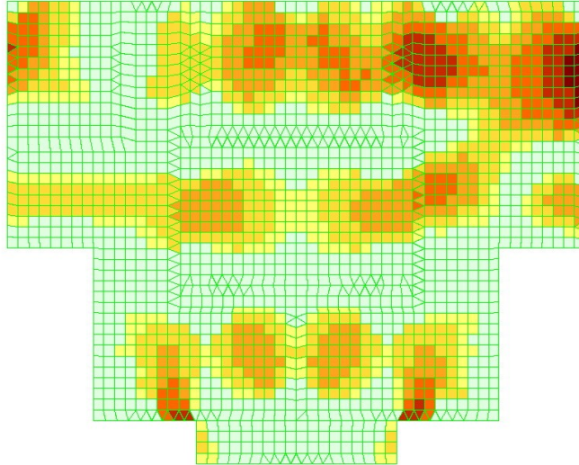
Рис. 7 – Изополя армования плиты перекрытия при розрахунку за допомогою побудови просторових елементів ґрунта (піщані ґрунти)
