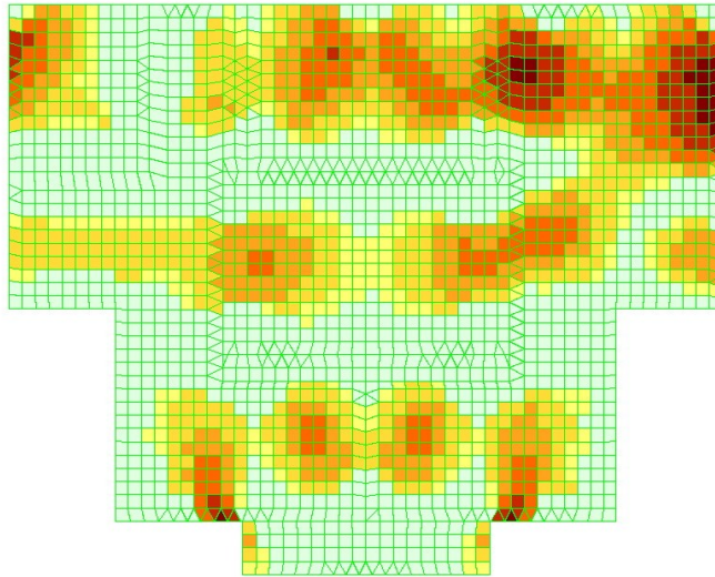
Рис. 6 – Изополя армования плиты перекрытия при розрахунку за допомогою коефіцієнтів постелі (глинисті ґрунти)
