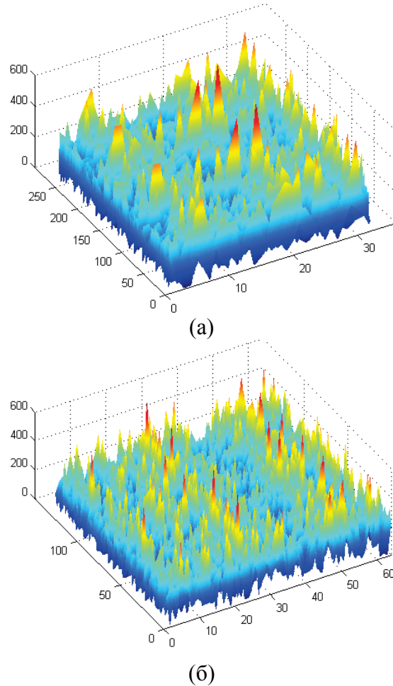
Рис. 1. Спектральні компоненти згенерованої ритмокардіограми (вісь абсцис — k , номер компоненти; вісь ординат — l \times 3 \cdot 10^{-3} , індекси гармонік спектру; Гц ; вісь аплікату — спектральна густина потужності, мс^2/Гц )
