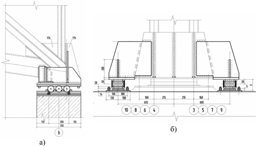
Рис. 4. Принципове рішення підсилення шарнірно-рухомих вузлів ферм парними додатковими опорами на циліндричних котках: а – виз збоку, б – задній вид.
