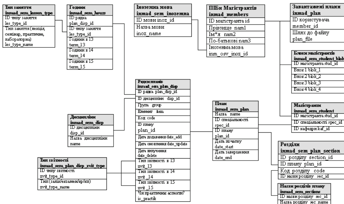
Рис. 2. Структура бази даних підготовки індивідуальних планів
