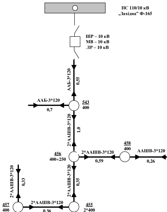
Рис. 2. Фрагмент спостережної електричної мережі 10 кВ
