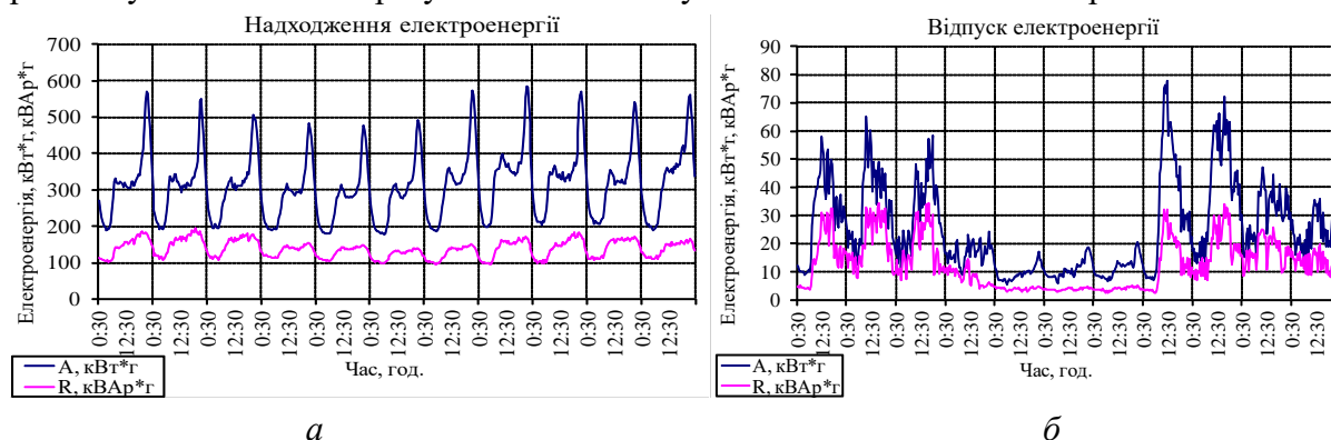
Рис. 3. Приклад вимірних значень протягом одинадцяти днів:
