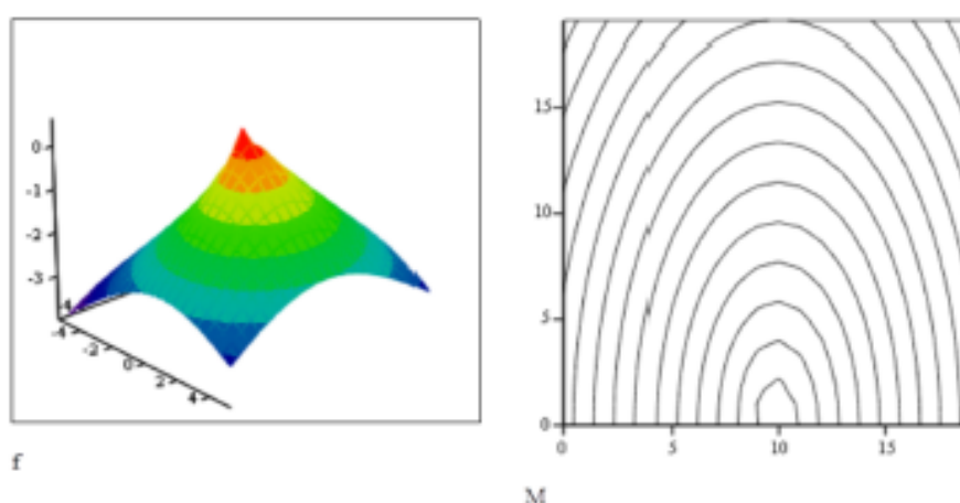
Рис. 2 Графік функції та лінії рівня.
