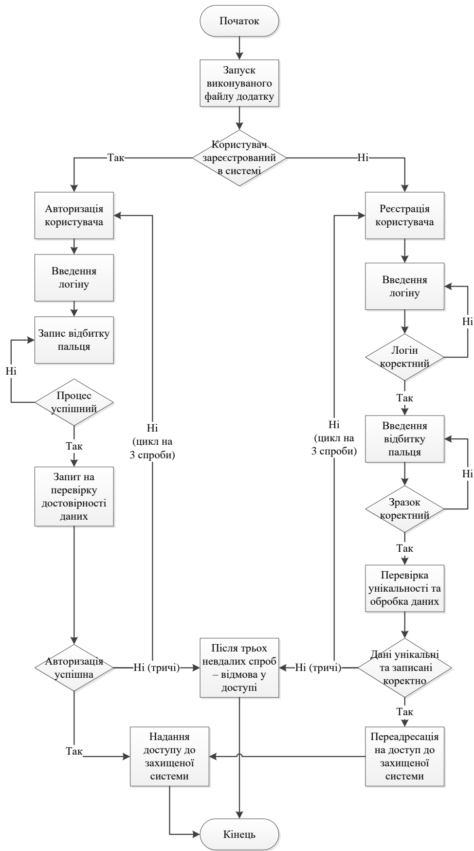
Рисунок 1. Блок-схема алгоритму роботи програмного додатку для автентифікації користувачів засобами вдосконаленої технології дактилоскопії
