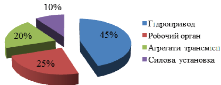
Рисунок 1 – Поширеність відмов агрегатів смiттевозів
