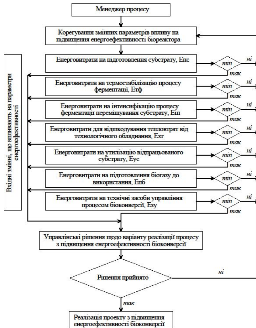
Рис. 4. Структурно-логічна модель управління проектом з підвищення енергоефективності процесу біоконверсії
