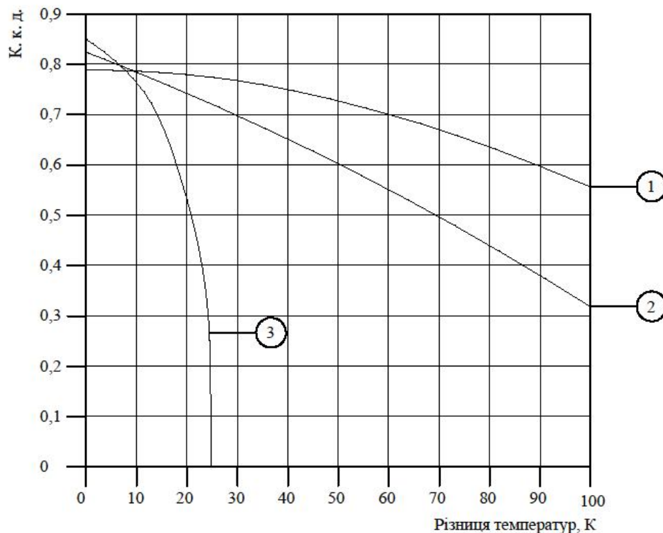
Рис. 5. Порівняння ККД сонячних колекторів
