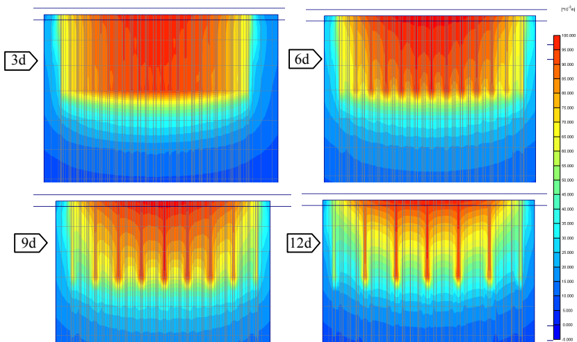
Рис. 2. Вертикальные перемещения грунта основания системы «ленточный свайный фундамент–основание» для свай длиной 9 м при разном продольном шаге свай
