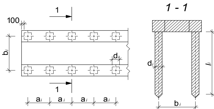
Рис. 1. Модель ленточного фундамента при усилении сваями
