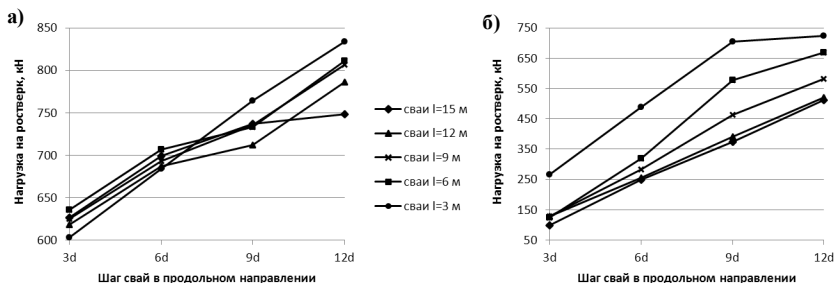
Рис. 3. Зависимость нагрузки, которая воспринимается ростверком, при различной длине свай от шага свай в продольном направлении для систем «ленточный фундамент мелкого заложения–сваи усиления–основание» (а) и «ленточный свайный фундамент–основание» (б)
