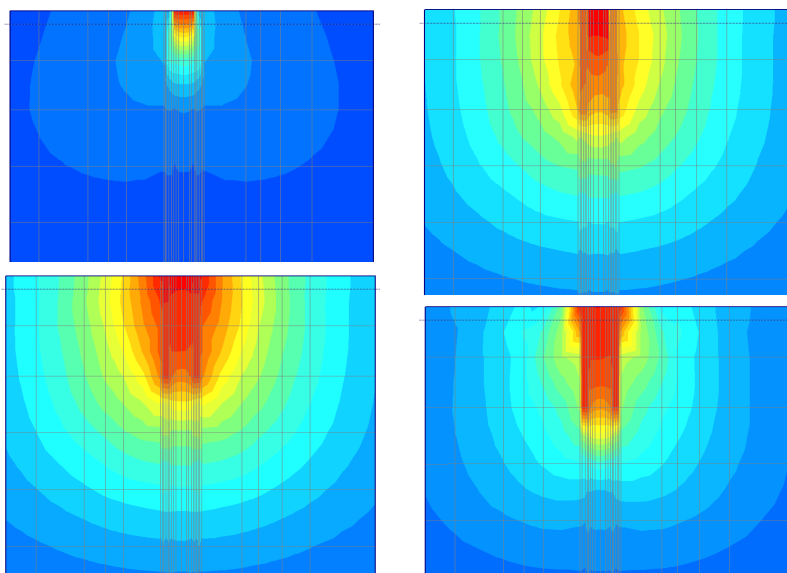
Рис. 3. Вертикальные перемещения грунта основания системы «ленточный фундамент мелкого заложения фундамент–сваи–основание» для свай длиной 6 м на разных этапах приложения нагрузки: а – ленточный фундамент мелкого заложения до усиления; б – устройство свай усиления; в – объединение свай усиления с существующим фундаментом; г – увеличение нагрузки
