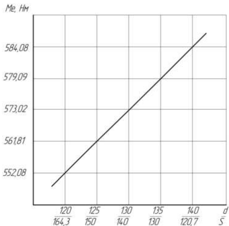
Рисунок 2 - Залежність максимального крутного моменту M_e від відношення діаметру поршня до його ходу дизельного двигуна ЯМЗ-238 де, кг/(кВт·год)
