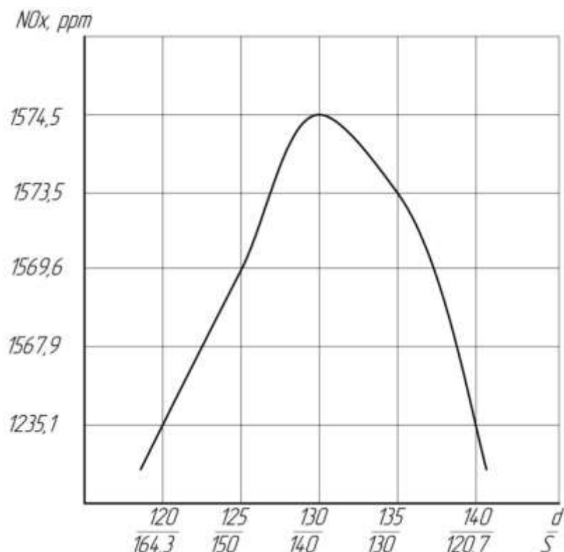
Рисунок 4 - Залежність викидів оксиду азоту NO_x від відношення діаметру поршня до його ходу дизельного двигуна ЯМЗ-238
