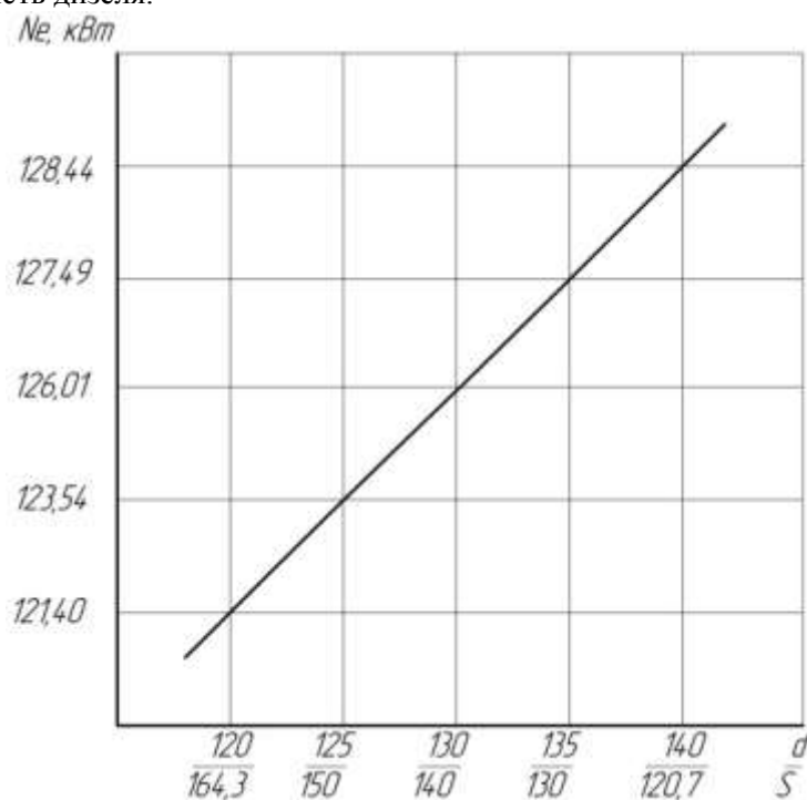
Рисунок 1 - Залежність номінальної потужності N_e від відношення діаметру поршня до його ходу дизельного двигуна ЯМЗ-238
