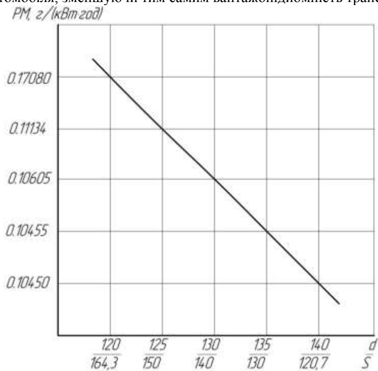
Рисунок 5 - Залежність емісії твердих часток від відношення діаметру поршня до його ходу дизельного двигуна ЯМЗ-238
