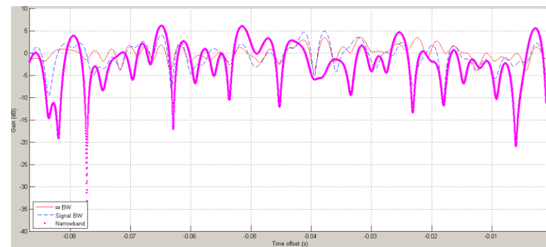
Рисунок 4 – Коефіцієнт підсилення багатопроменевих складових прийнятого сигналу
