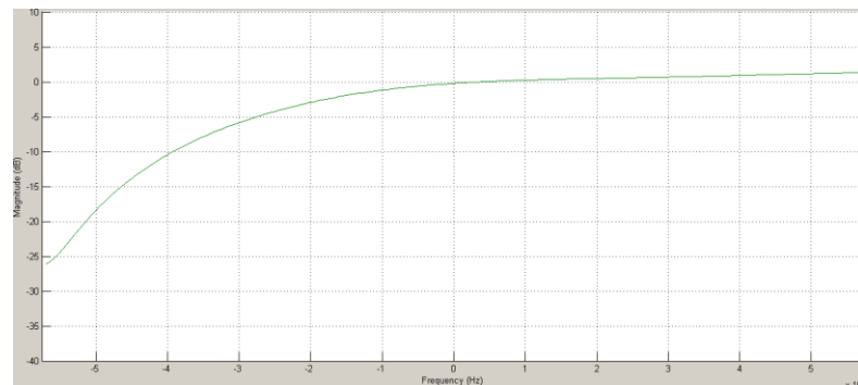
Рисунок 2 – Частотна характеристика мережі
