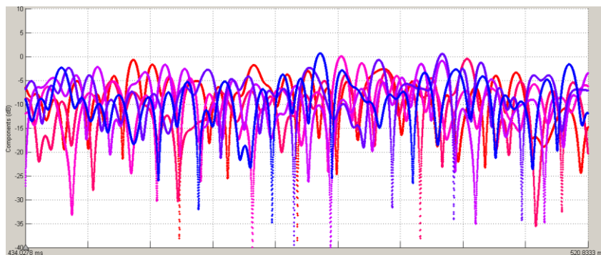
Рисунок 3 – Багатопроменеві згасаючі складові прийнятого сигналу
