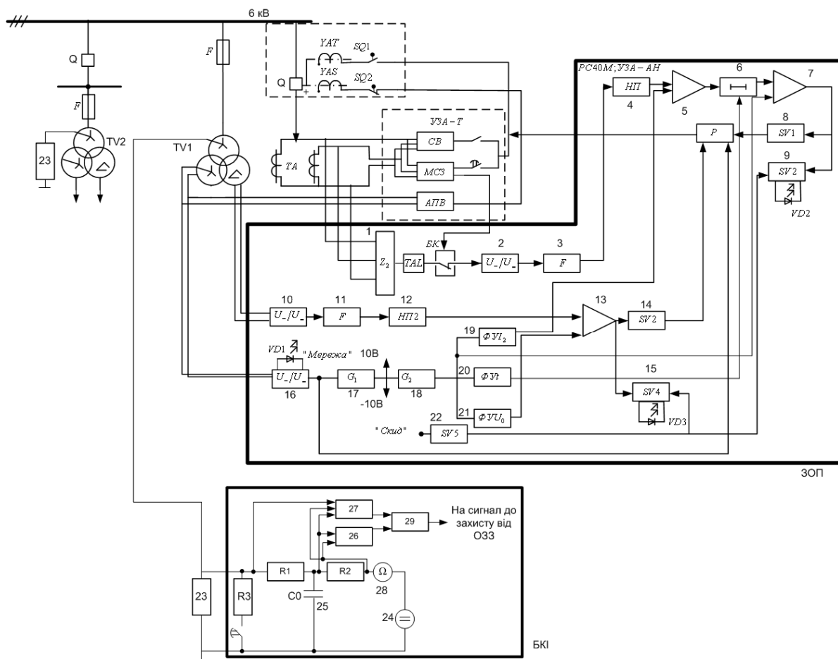
Рисунок 1 – Функціональна схема комбінованої системи протиаварійної автоматики
