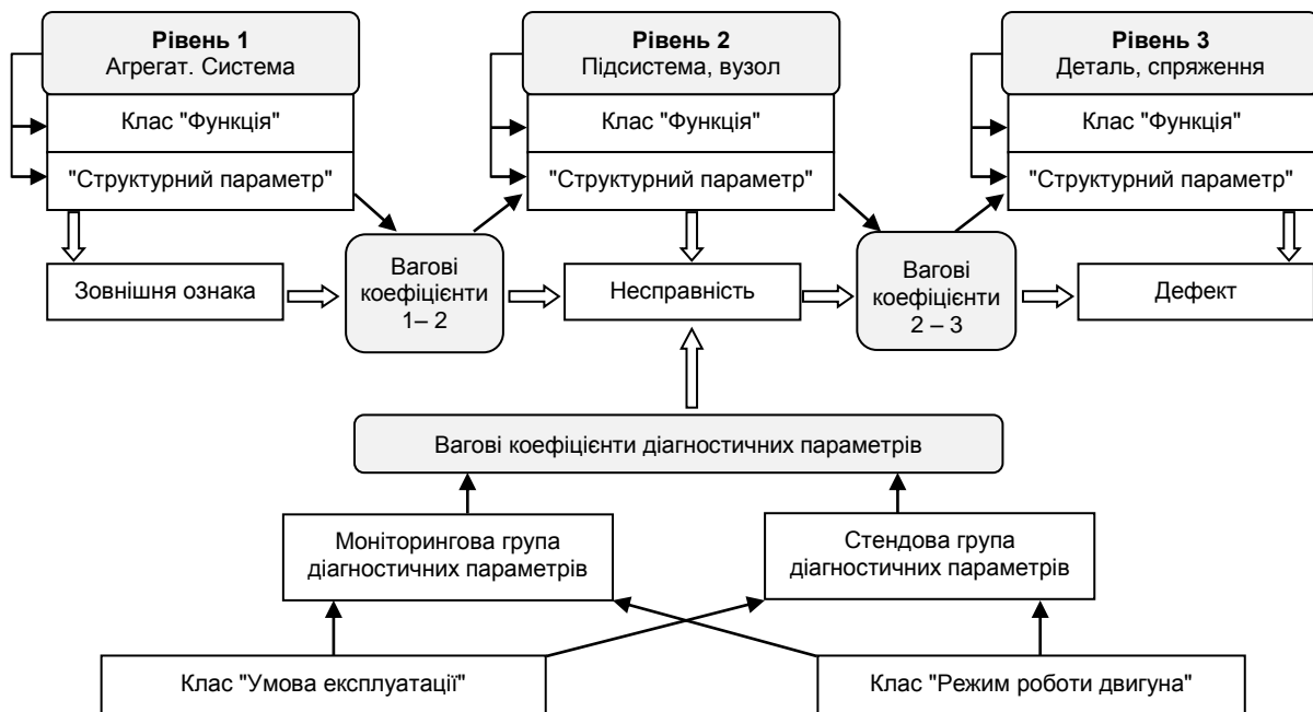
Рис. 1. Загальна схема ідентифікації технічного стану
