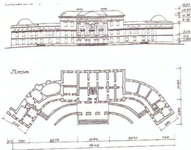
Рис. 1. План та фасад палацу Можайського
