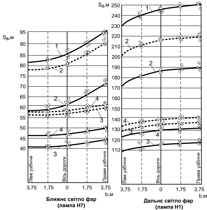
Рис. 5. Експериментальна залежність дальності видимості від характеристик об'єкта розрізнення для фар з лампами Н7, Н1 (Opel Astra G): 1 - тест-об'єкт (загальна видимість); 2 - тест-об'єкт (пішохід) у світлому одязі; 3 - тест-об'єкт (пішохід) у темному одязі; 4 - тест-об'єкт (пішохід) у одязі зі світловідбиваючими елементами; — - дальність конкретної видимості; ..... - дальність силуетної видимості, S_b - дальність видимості; b - ширина дорожнього полотна
