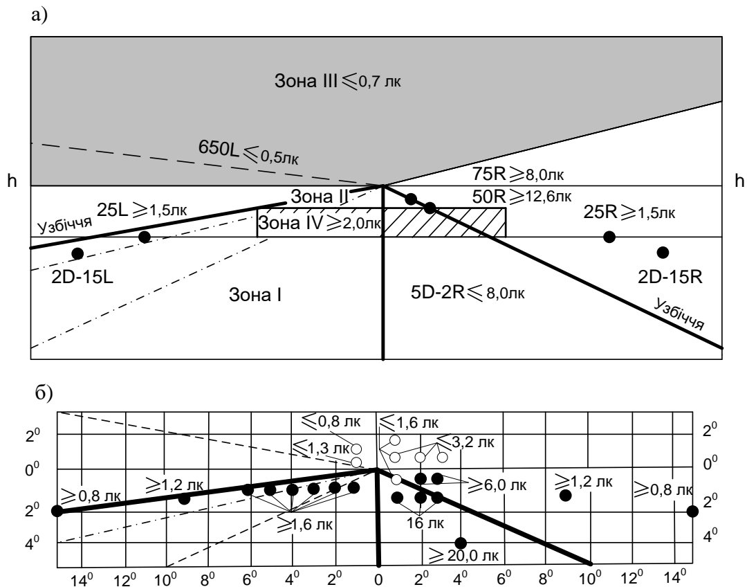
Рис. 3. Перспектива двополюсної дороги (а) і вимірювальний екран (б): ○ - точки, у яких обмежується верхня границя сили світла; ● - точки, у яких обмежується нижня границя сили світла
