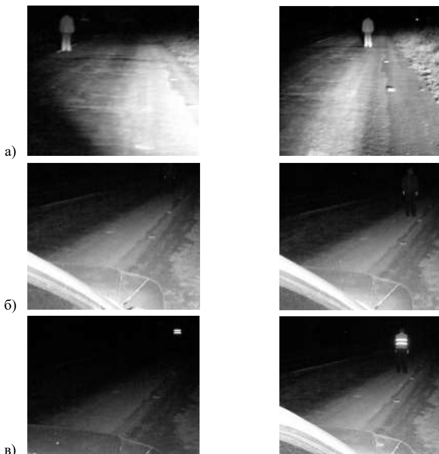
Рис. 4. Проведення експериментів з визначення величини дальності видимості (силуетної та конкретної), враховуючи колір та особливості одягу пішохода, тип і стан дорожнього покриття
