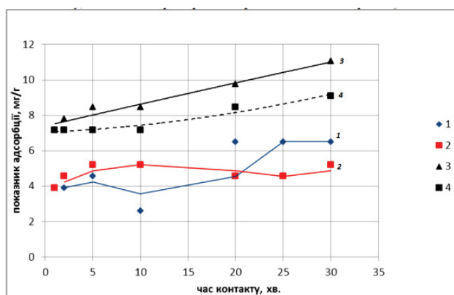
Рис. 1 Вплив температури на швидкість процесу адсорбції іонів цинку на активованих лугом (3, 4) і природних (1, 2) глинистих зразках при температурах 285 К (2, 4) і 328 К (1, 3)
