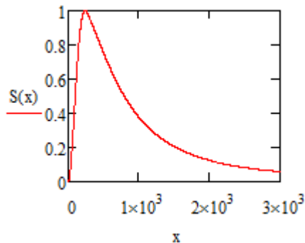
Рисунок 1.3 - Графік концентрації оксиду карбону в повітрі від відстані від джерела викиду
