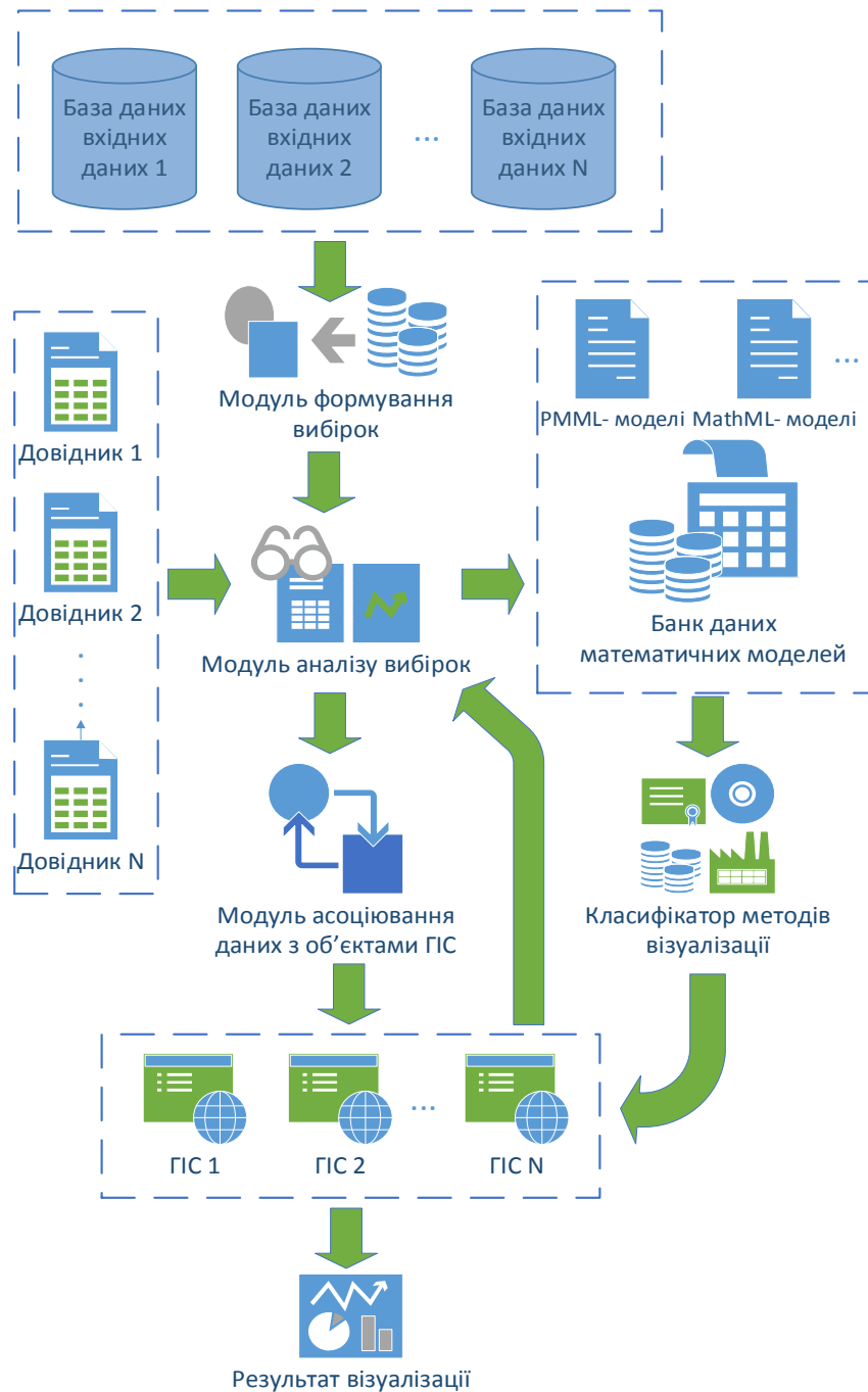
Рис. 1. Структура ГІС-інтегрованої системи даних та моделей на основі XML-формалізації
