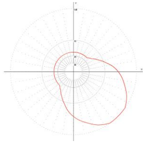
Розрахункова діаграма спрямованості антени
