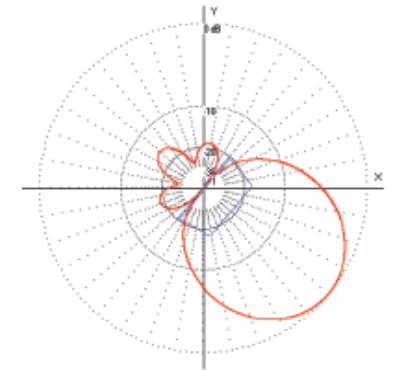
Діаграма спрямованості випромінювання відповідно виконанню проекту
