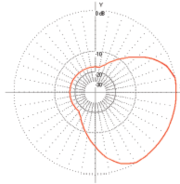
Діаграма спрямованості випромінювання відповідно рекомендацій регуляторного органу
