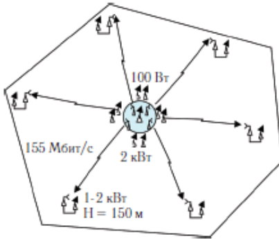
Схема ідеальної типової SFN мережі для портативного прийому
