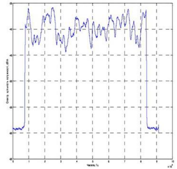
Спектр сигналу в райсівському каналі
