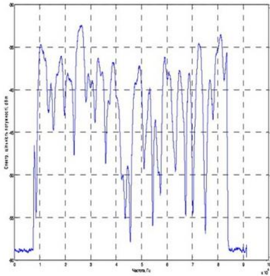
Спектр сигналу в релеєвському каналі
