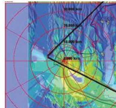
Результати розрахунків зони покриття передавальної станції
