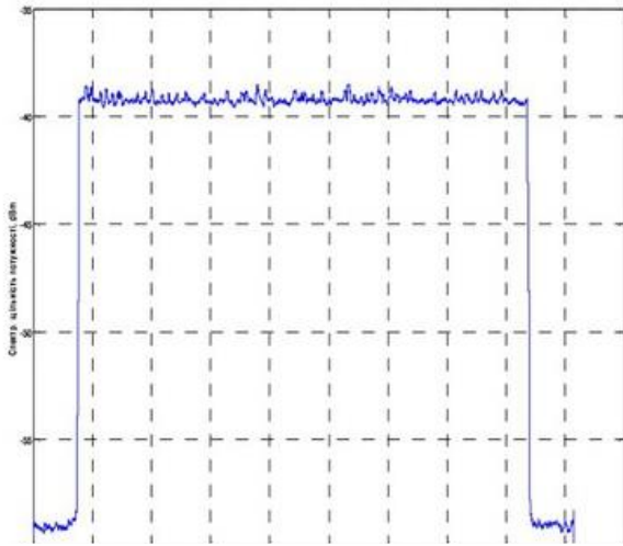
Спектр сигналу в AWGN каналі
