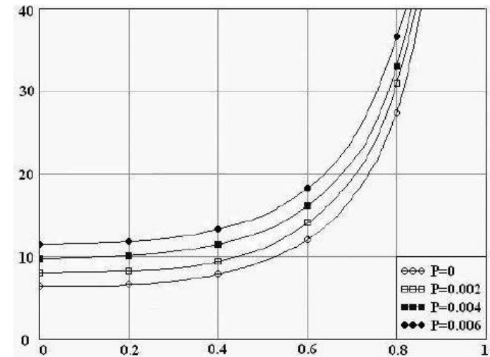
Залежність часу затримки пакетів в висхідному каналі від інтенсивності вхідних навантаження при зміні ймовірності бітових помилок
