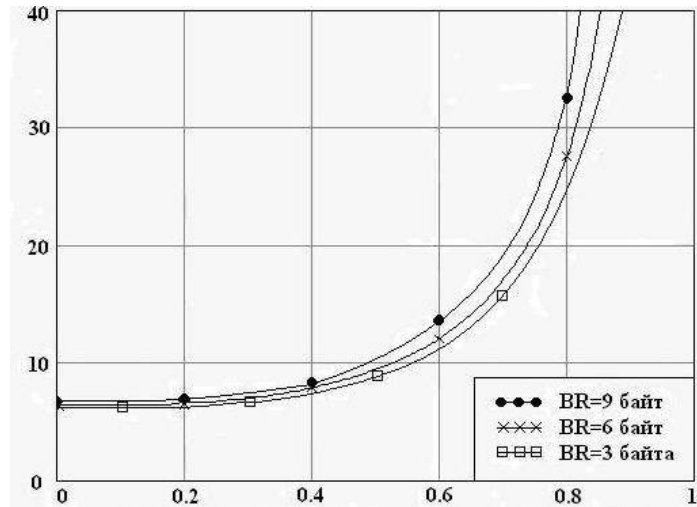
Залежність часу затримки пакетів в висхідному каналі від інтенсивності вхідних навантаження при зміні розміру запиту смуги пропускання
