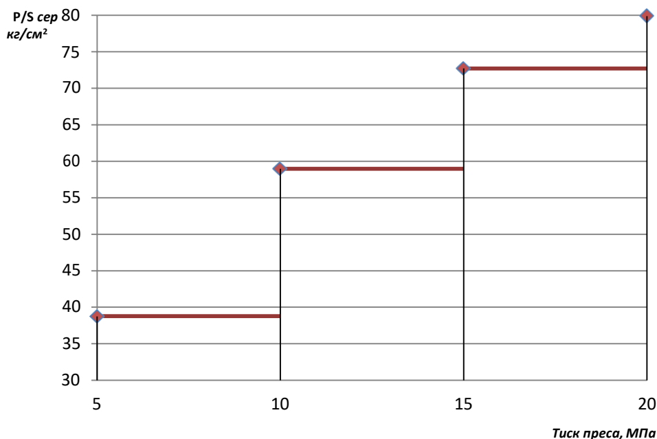
Рис.2 Залежність середньої граничної міцності від тиску пресування
