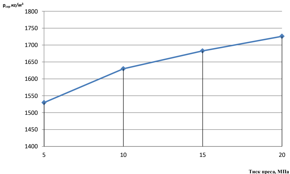
Рис.1 Залежність залежності середньої густини від тиску пресування.
