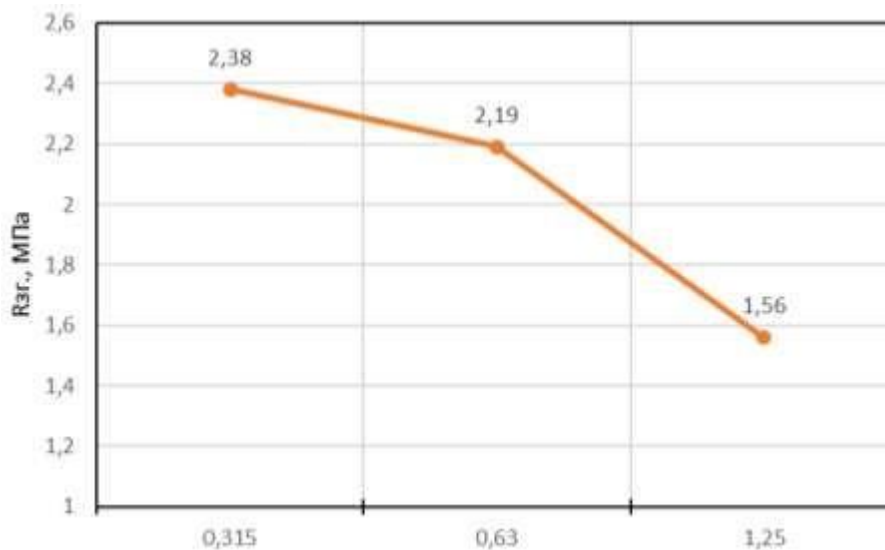
Рис. 2. Залежність міцності на згин СБС від granulometрії мінеральних наповнювачів
