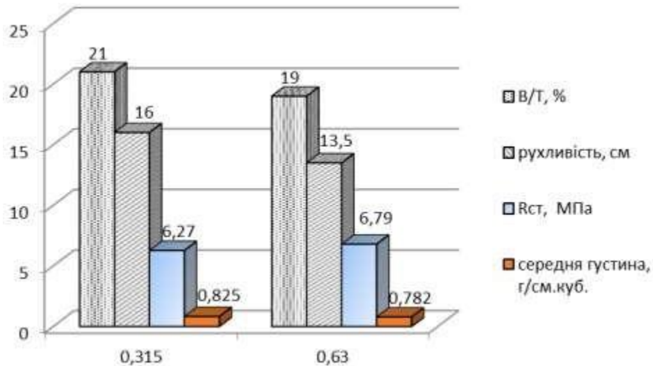
Рис. 3. Залежність властивостей СБС з полімерними добавками від гранулометрії мінеральних наповнювачів
