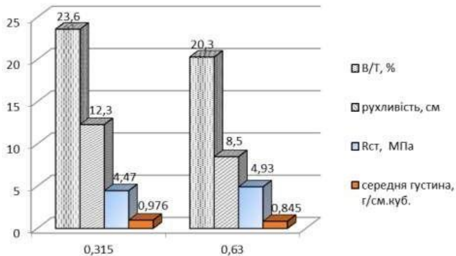
Рис. 1. Залежність властивостей СБС від granulometрії мінеральних наповнювачів
