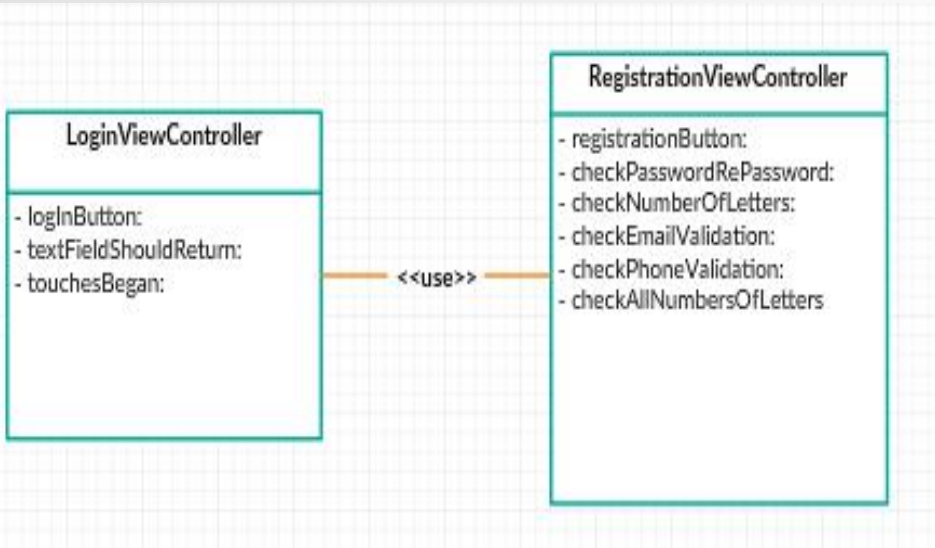
Classes Diagram of the module «User Authorization» Registration
