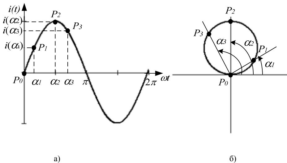
Рис. 2. Представлення змінного струму: а) — в прямокутних; б) — полярних координатах
