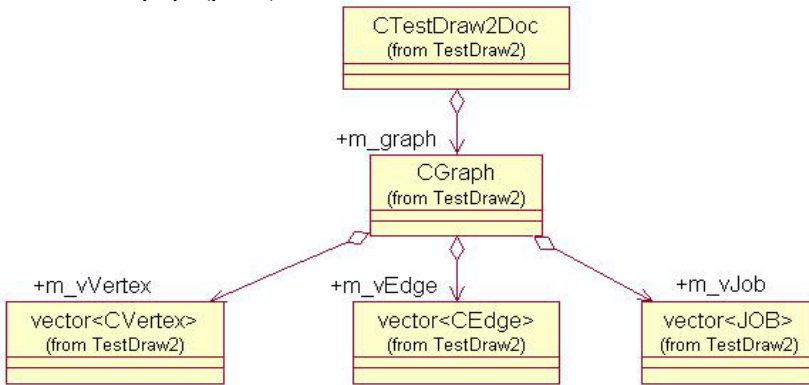
Рисунок 1 – UML-діаграма реалізації класу графічного представлення графа
