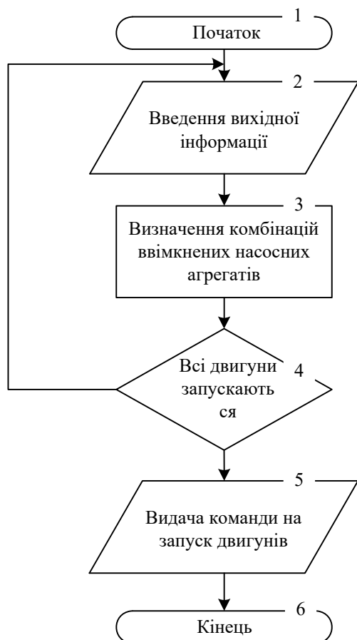
Рисунок 1 – Алгоритм автоматизованого запуску двигунів насосних агрегатів при їх паралельній роботі
