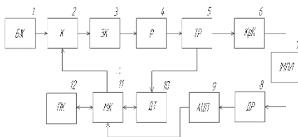
Рис. 1. Структурна схема пристрою тестування імплантатів.
