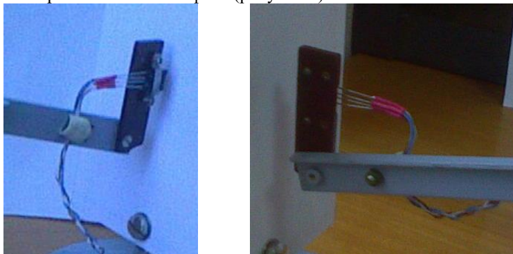
Рис. 2. Тримач оптопарі
