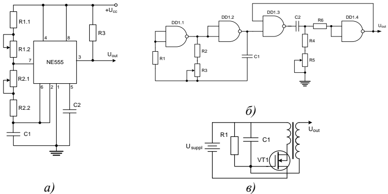
Рис. 1 – Варіанти схем генераторів холодної плазми: а) класична схема на таймері NE555; б) генератор на логічних елементах; в) блокінг-генератор Література
