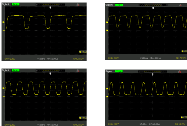
Рис. 2 – Приклади форм вихідного сигналу тахометричного перетворювача на базі відбивної оптипари
