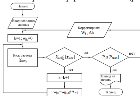
Рис. 2. Укрупненная блок-схема алгоритма автоматизированного проектирования технологических режимов работы и настройки оборудования косоваляковых трубоправильных машин.
