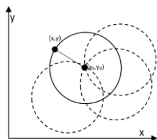
Рис. 2. Розпізнавання окружності методом Хафа
