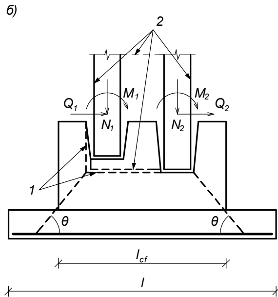
Рисунок 8.2 – Утворення піраміди продавлювання від двох колон: – розміщення колон в одному рівні; б – розміщення колон в різних рівнях; 1 – внутрішня грань стакана; 2- зовнішня грань умовної колони
