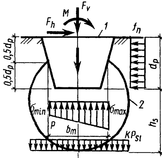
Рисунок 6.3 – Схема до розрахунку стовпчастого фундаменту у витрамбуваному котловані
