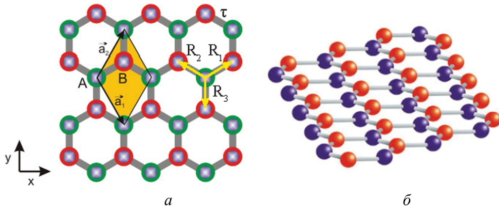
Рис. 2. Структура графена: a – атомная структура графена состоящая из гексагонов с расстоянием между атомами AB=1,42\text{E} и параметрами подрешеток a_1, a_2 = 2,46\text{E} ; б – кристаллографическая структура графена состоит из двух эквивалентных подрешеток А (красные) и В (фиолетовые) атомов, которые образуют двумерную плоскость с двумя энергетическими зонами левого и правого спинов (хиральностью)
