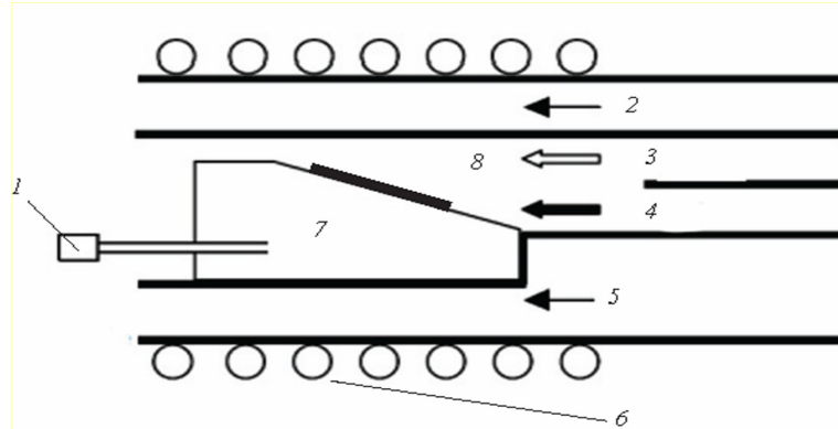
Рис. 1. Схематическое изображение горизонтального MOCVD-реактора, 1-термопара, 2,5-обходной поток азота, 3-поток аммиака, 4-поток триметилалюминия, 6 – индукционный нагрев, 7- подложкодержатель, 8-подложка
