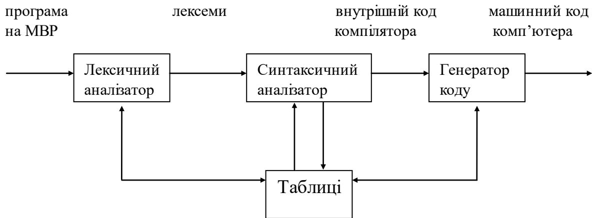
Рис.1.6. Спрощена модель компілятора
