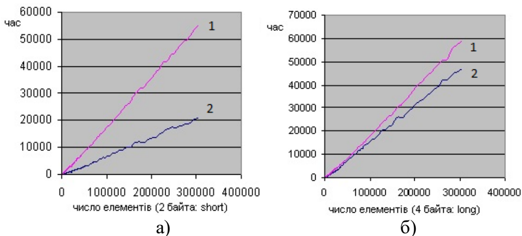
Рис. 2.7. Результати порівнянь швидкого сортування (лінія 1) і порозрядного сортування (лінія 2): а) тип даних short; б) тип даних long.
