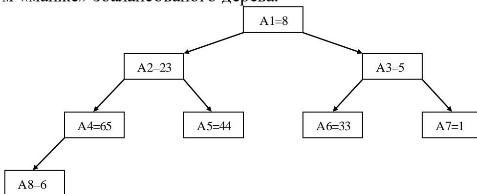
Рис. 2.5. Деревовидне представлення масиву
