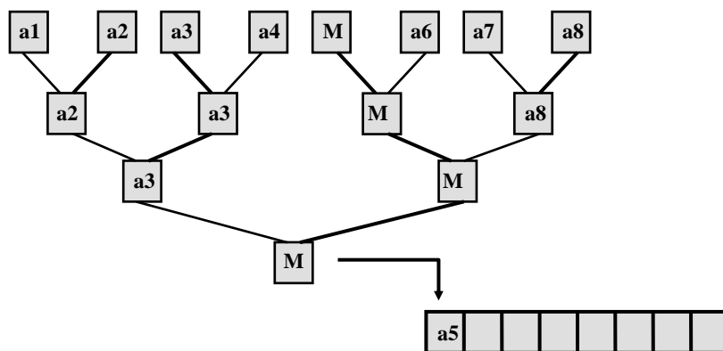
Рис.2.2. Приклад сортування деревом (мінімальний елемент пересилається у вихідний масив B )
