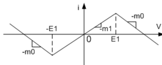
Рисунок 3 – Вольт-амперна характеристика нелінійного резистора
