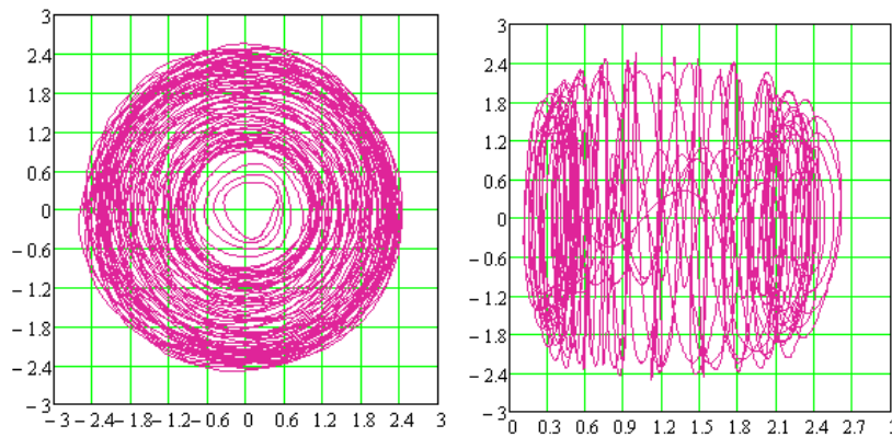
Рисунок 5 – Проекція на площину \{V_{C1}, V_{C2}\} при \alpha = 2
