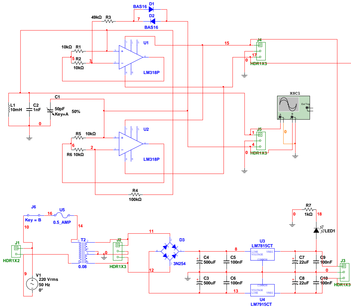
Рисунок 4 – Реалізація схеми (рис. 2) в пакеті схемотехнічного моделювання MultiSim
