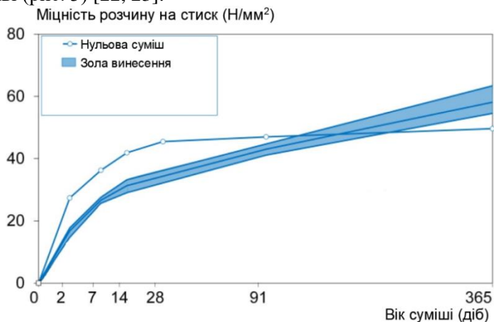
Рисунок 3 – Графік залежності зміни міцності бетонної суміші протягом року з додаванням золи винесення і без
