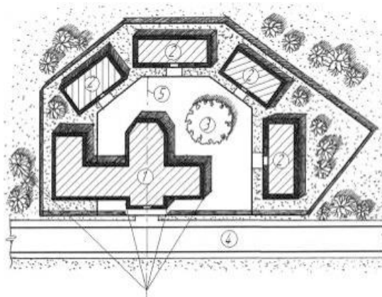
Рис. 5. Схема „вільного” розвитку генплану
