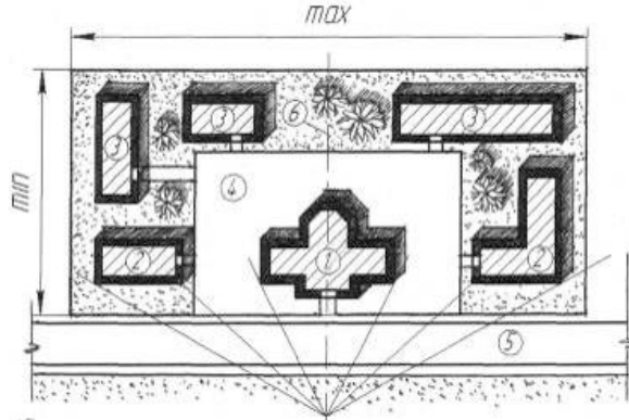
Рис. 4. Схема „фронтального” розвитку генплану
