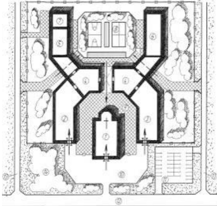
Рис. 1. Схема генплану духовно-освітнього комплексу із загальнодоступним храмом
