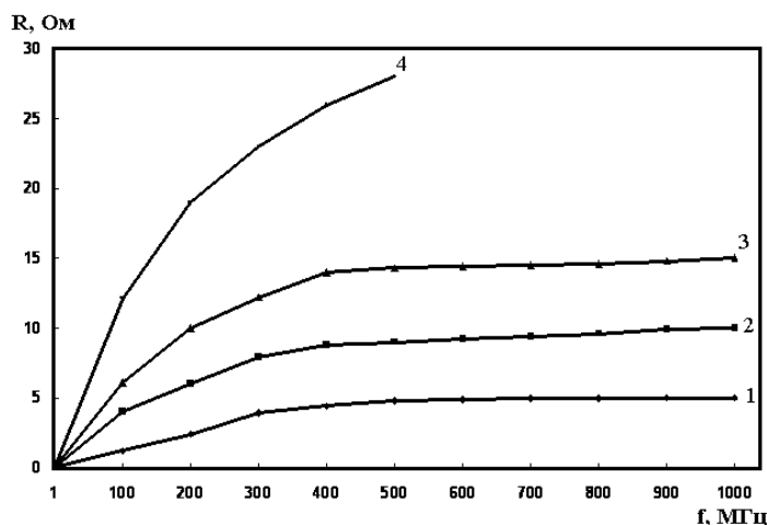
Рис. 5. Теоретичні залежності активної складової імпедансу каналу від частоти при T=\text{const}, U_3=\text{const} : 1– T=188\text{ K}, U_3=4\text{ В} ; 2– T=373\text{ K}, U_3=4\text{ В} ; 3– T=188\text{ K}, U_3=3\text{ В} ; 4– T=373\text{ K}, U_3=3\text{ В}
