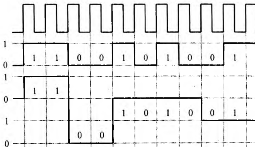
Рисунок 4 — Схема кодування PAM
