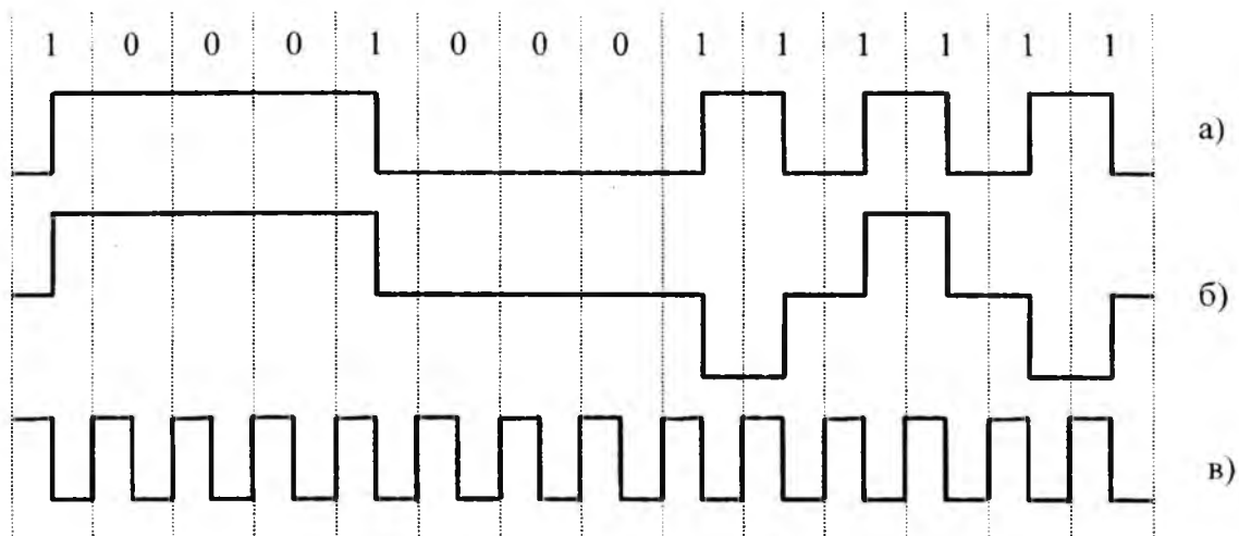
Рисунок 3 — Схема кодування MLT-3: а) сигнал у кодї NRZI, б) сигнал у кодї MLT-3, в) сигнал тактового генератора
