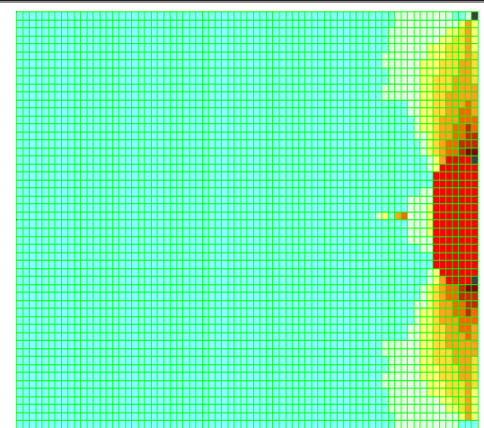
Площадь арматуры на 1м по оси Y у верхней грани; максимум в элементе 1875
