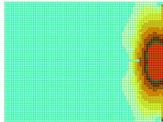
Площадь арматуры на 1м по оси X у верхней грани; максимум в элементе 1439
