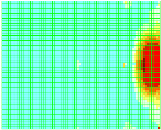
Площадь арматуры на 1м по оси X у нижней грани (балка-стена - по среднему); максимум в элементе 3719
