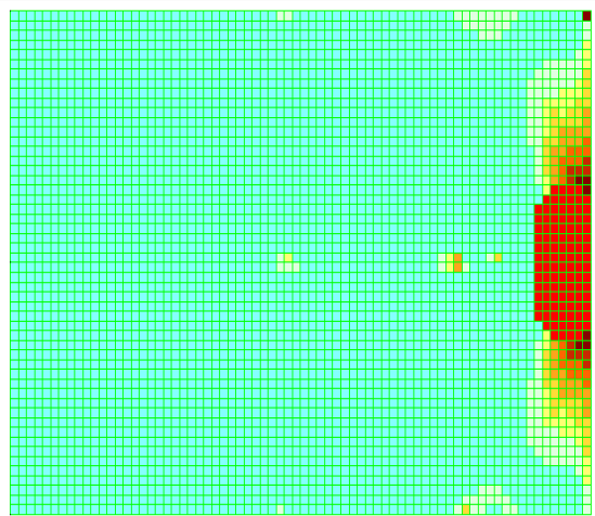
Площадь арматуры на 1м по оси Y у нижней грани (балка-стена - по среднему); максимум в элементе 3712
